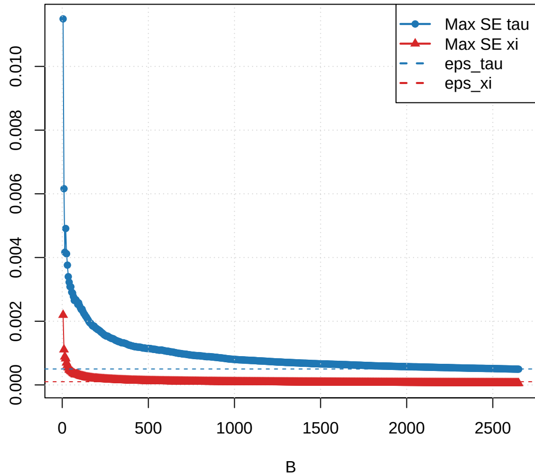
Max SE
